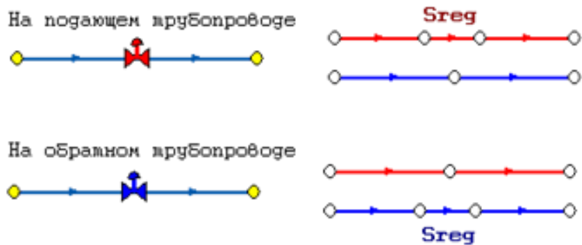
Рисунок 3.18 Дросселирующие устройства
